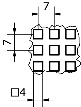
A (1:1) WZÓR PERFORACJI
