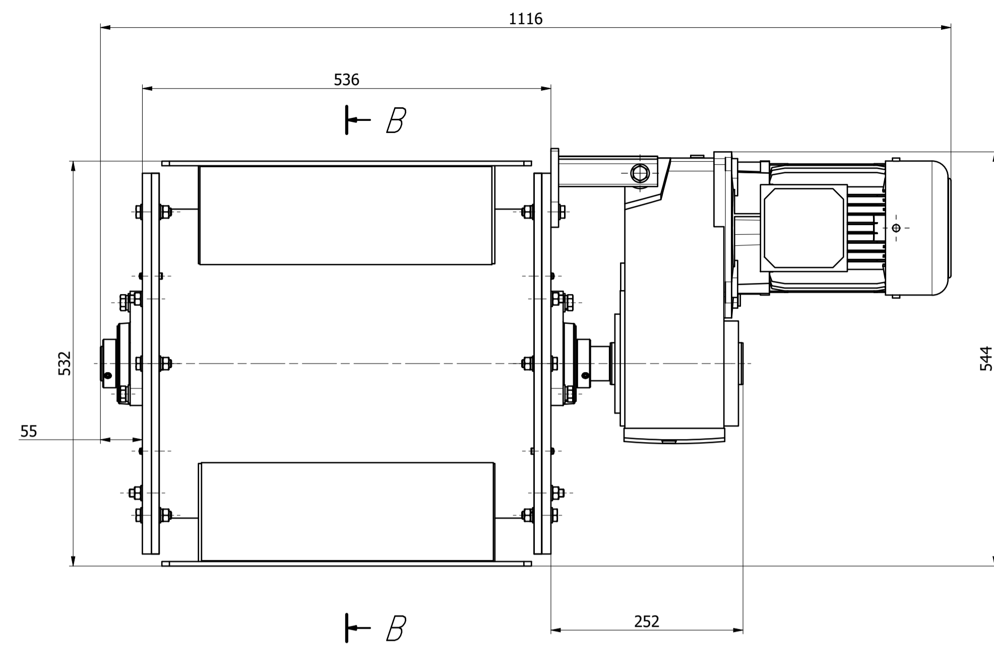
A-A (1:5)
